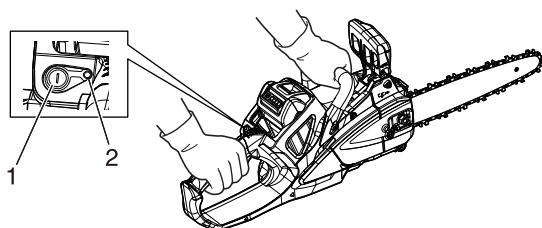
1. Strömbrytarknapp 2. Strömindikator diod
