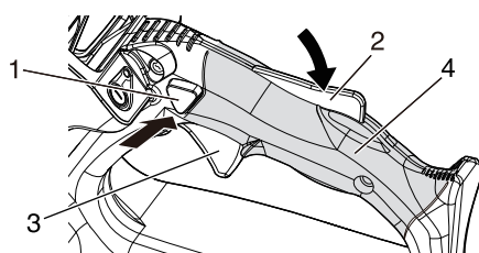
1. Avtryckarlås 3. Avtryckare 2. Frigöringsspak avtryckarlås
