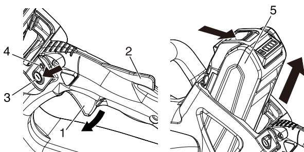
1. Avtryckare 4. Strömindikator diod 2. Frigöringsspak avtryckarlås 5. Batteri 3. Strömbrytarknapp
